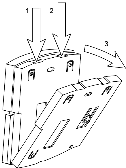
Рисунок 3 Демонтаж основания
