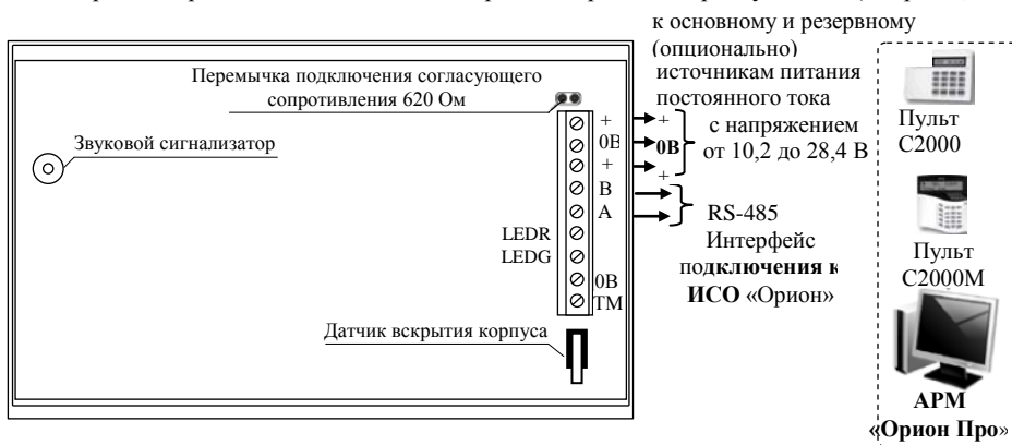
Рисунок 3. Схема внешних соединений блока
