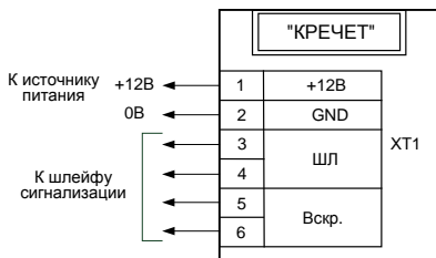
Рисунок 2 Схема подключения извещателя «Кречет»
