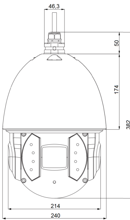
Рисунок 5.1 – Габаритные размеры видеокамеры (мм)
