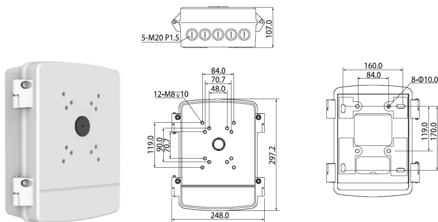
Рисунок 5.8 – Монтажная коробка BR-203
