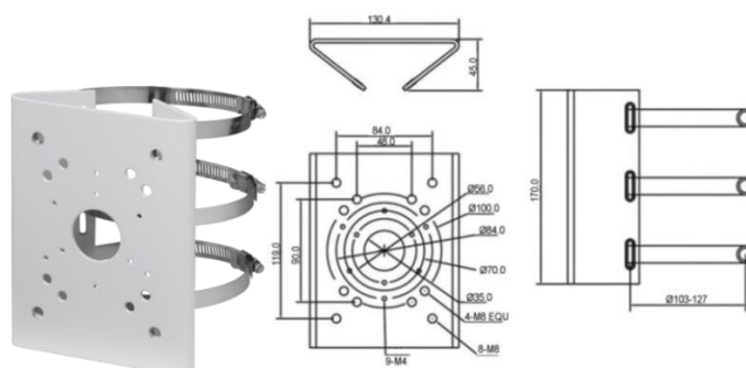
Рисунок 5.15 – Столбвой кронштейн BR-103
