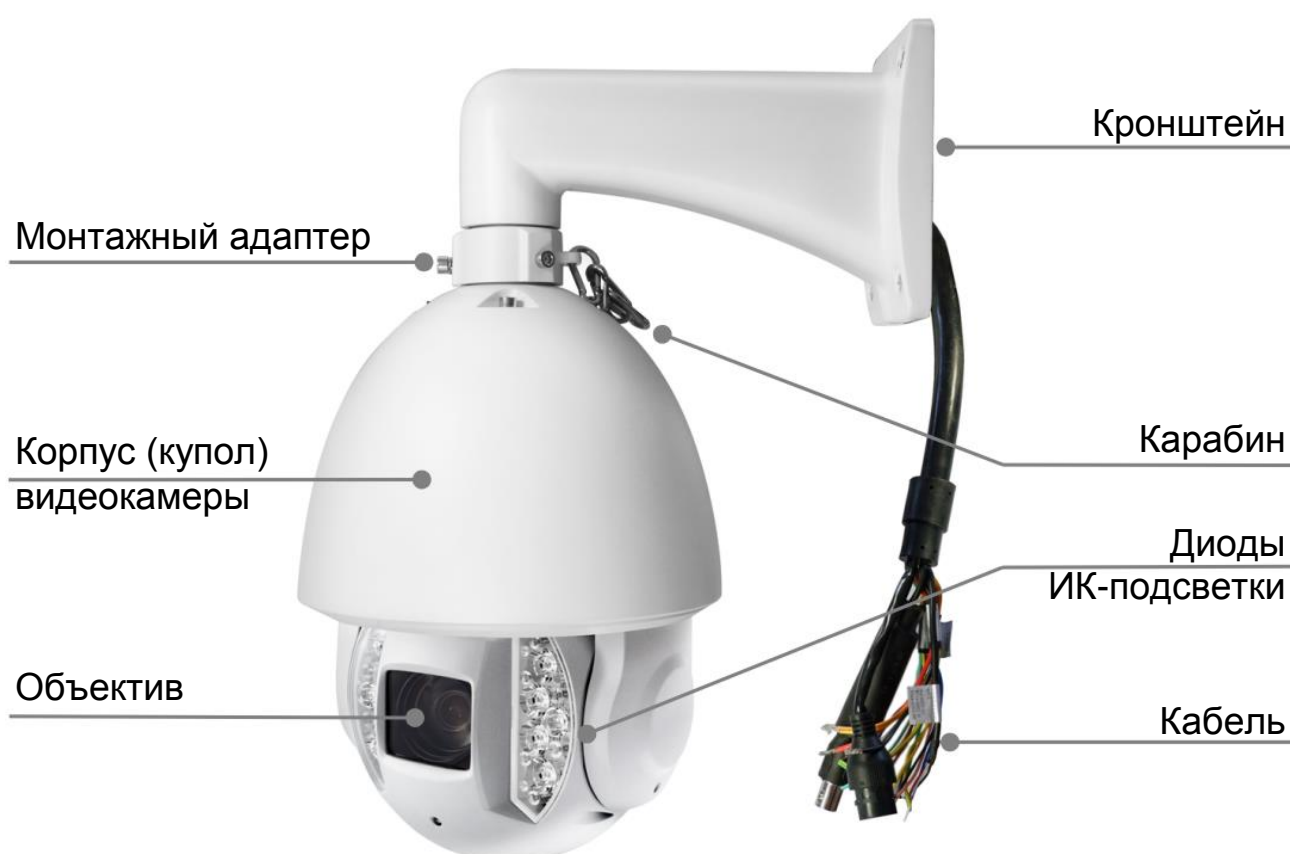
Рисунок 4.1 – Внешний вид и основные элементы видеокамеры
