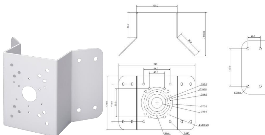
Рисунок 5.12 – Угловой кронштейн BR-102
