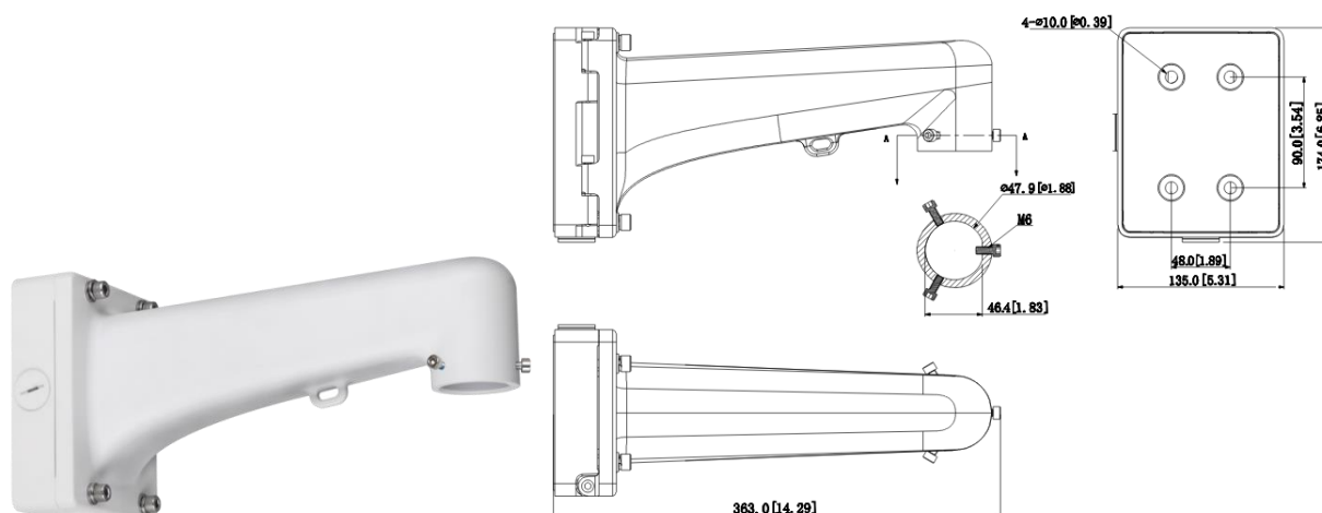
Рисунок 5.10 – Настенный кронштейн BR-110
